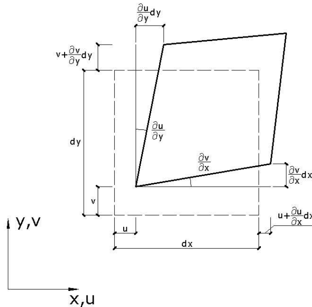
Rys. 6.2. Przemieszczenia i odkształcenia dla elementu płaskiego
