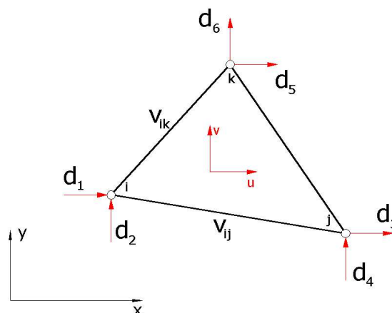
Rys. 6.3. Trójwęzłowy element trójkątny i definicja stopni swobody
