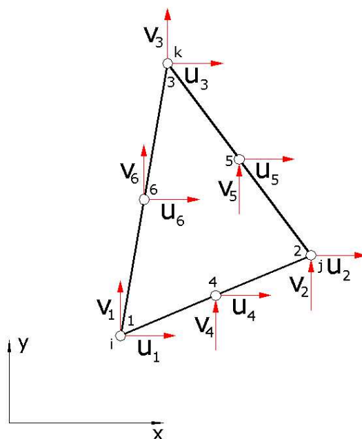
Rys. 6.4. Sześciowzłowy element trójkątny
